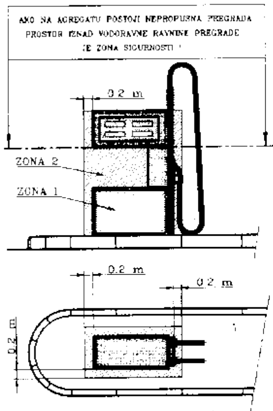
ZONE OPASNOSTI AGREGATA ZA TEKUĆA GORIVA
