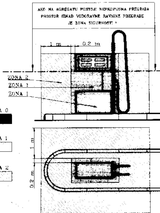
ZONE OPASNOSTI AGREGATA ZA UKAPLJENI NAFTNI PLIN
